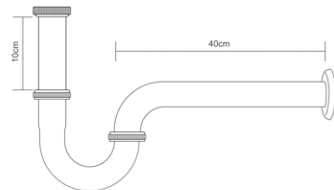
LX-P04 Drain-Pipe SUS304 Chrome
