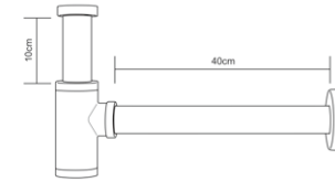
LX-P06 Drain-Pipe SUS304 Chrome
